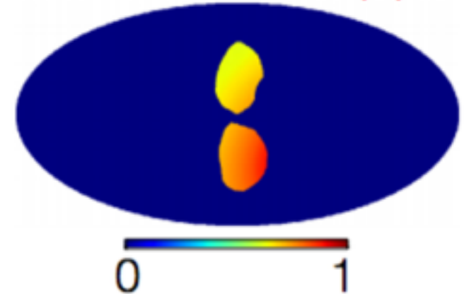
Fermi bubbles (1)
